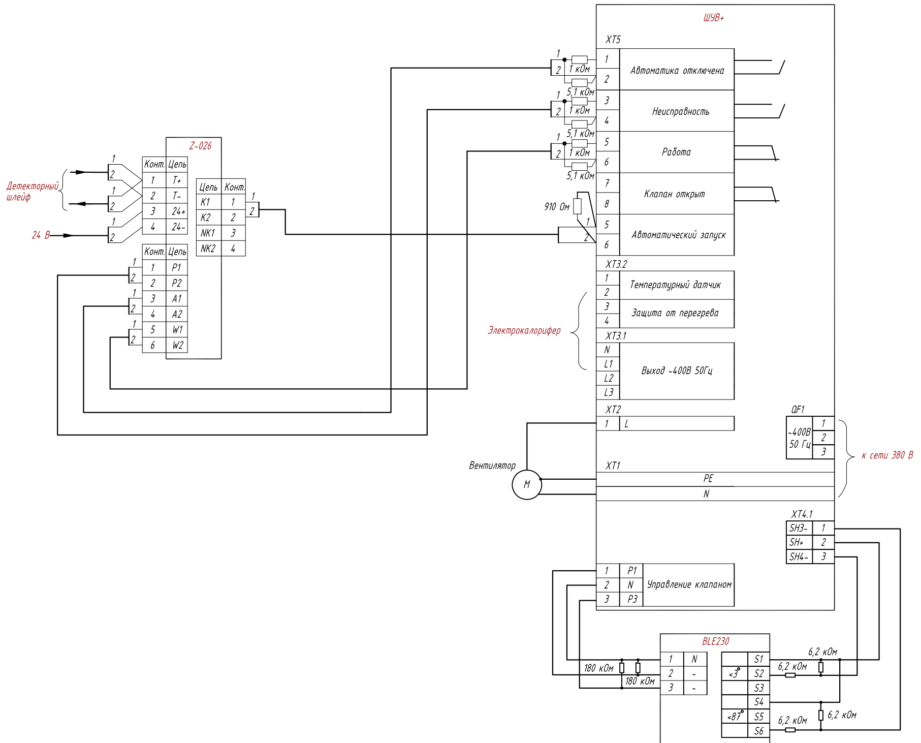
Схема подключения шкафа управления вентиляторами противодымной защиты серии ШУ типа ШУВ+. Схема внешних подключений для управления одним вентилятором 220В, одним реверсивным клапаном 220В и электрокалорифером 380В.
